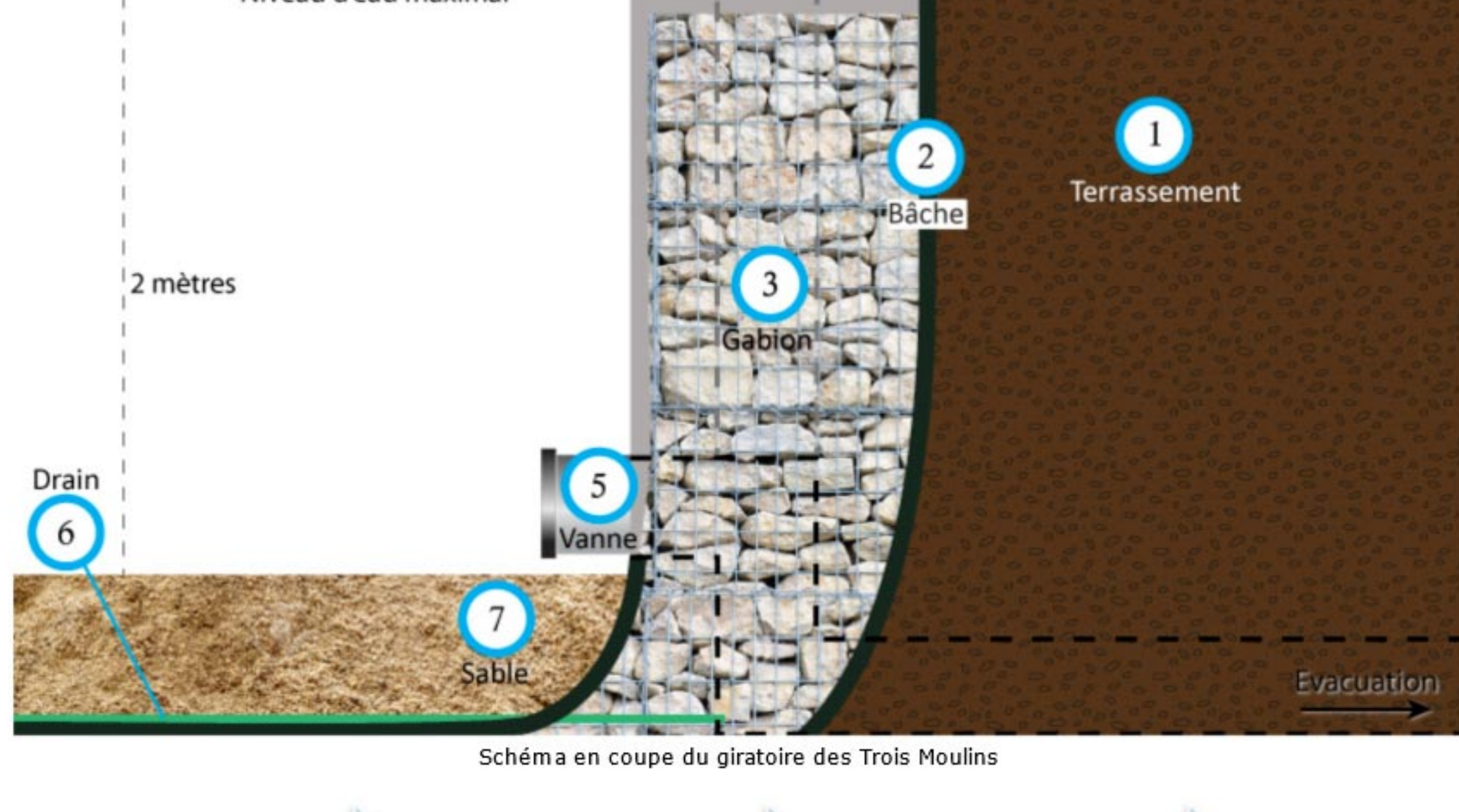
Schéma en coupe du giratoire des Trois Moulins
