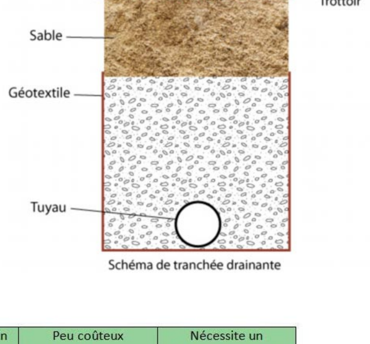
Schéma de tranchée drainante
